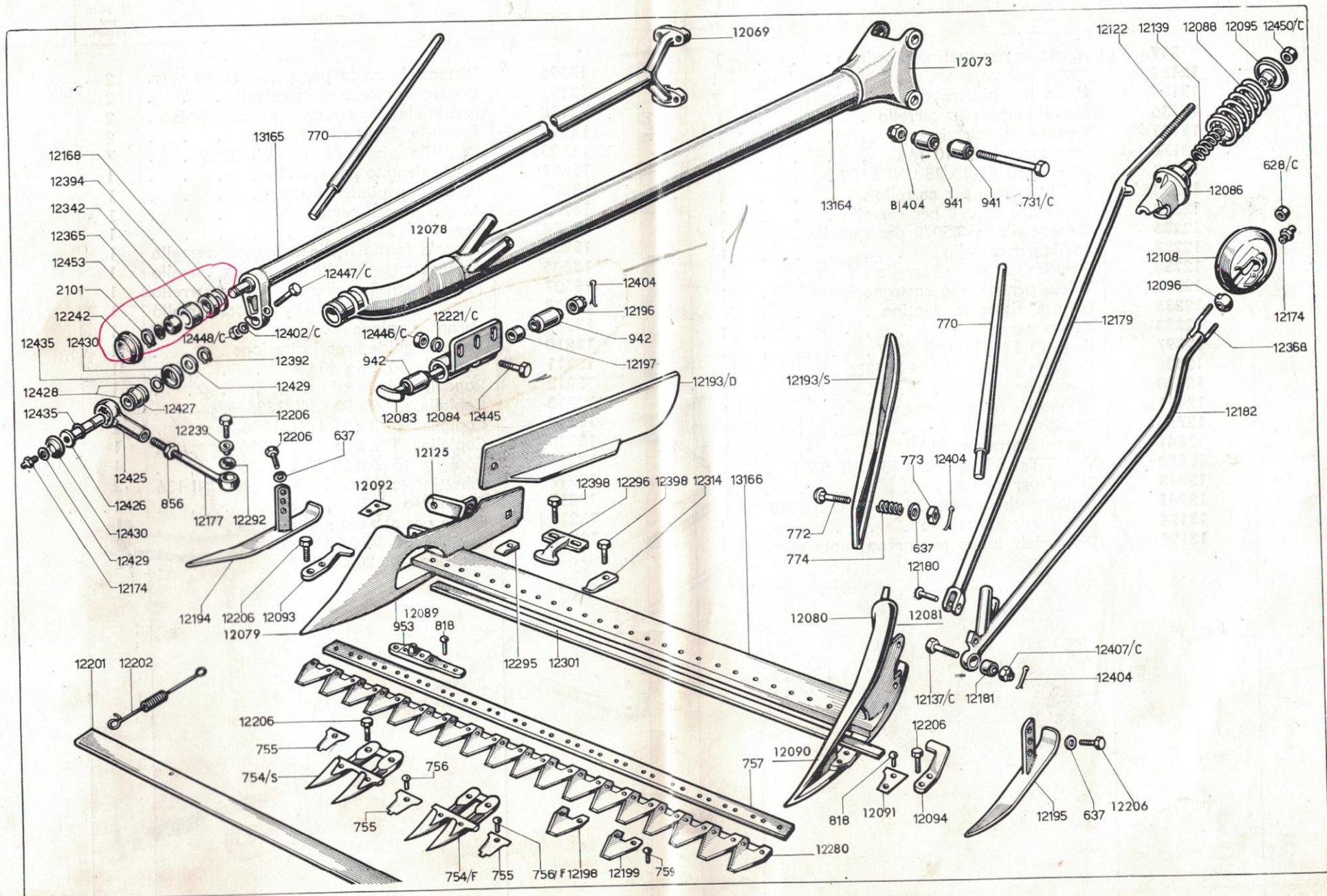
MOTOFALCIATRICE « OLYMPIA » TAV. 5
