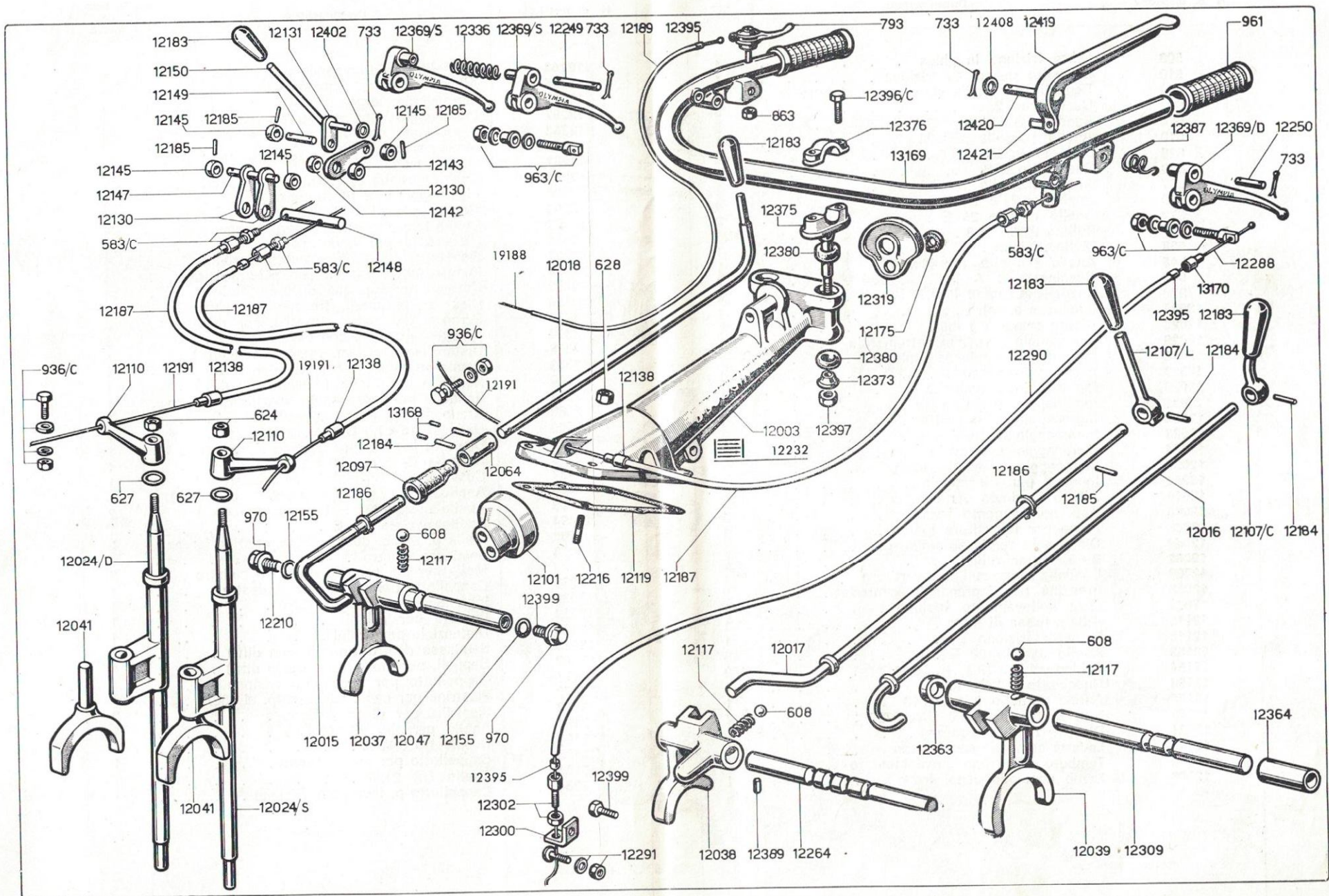
MOTOFALCIATRICE « OLYMPIA » TAV. 2
